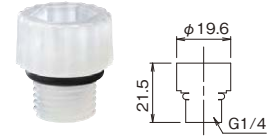
UPドレインプラグ(EPDM) 3C-S118000 見積価格 1/100 ●Oリング:EPDM
