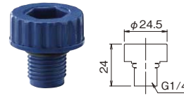
UHドレインプラグ(EPDM) 3C-S118005 見積価格 1/100 ●Oリング:EPDM
