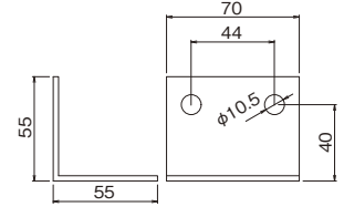
R2ブラケット 3C-2910 見積価格 1/20 ●材質:SUS304 ●UH・UP共用
