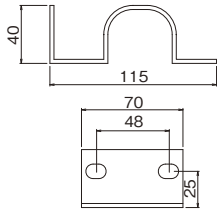
R3ブラケット 3C-2920 見積価格 1/20 ●材質:SUS304 ●UH・UP共用
