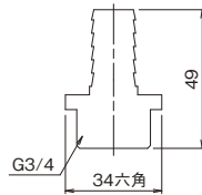
PPホースニップルセット 3C-3010 見積価格 1/50 ●材質:PP樹脂 ●UH・UP共用
