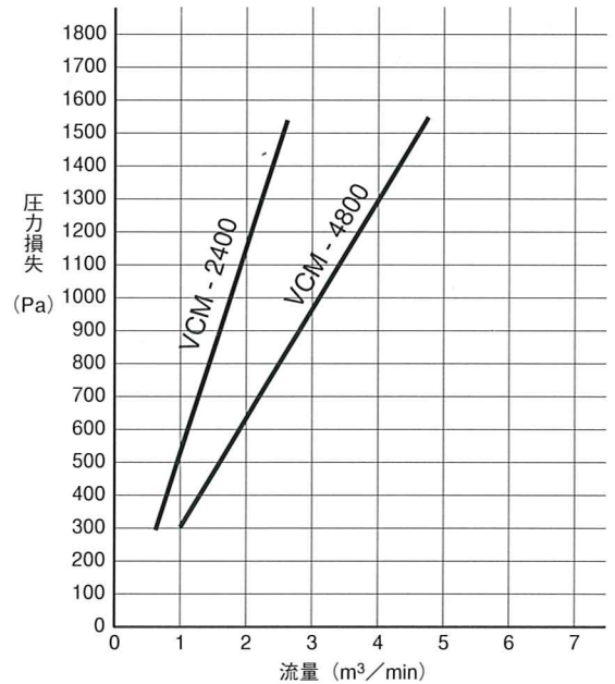
流量表
